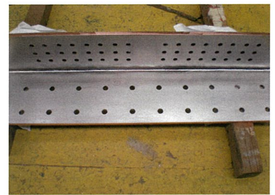
銅端子
