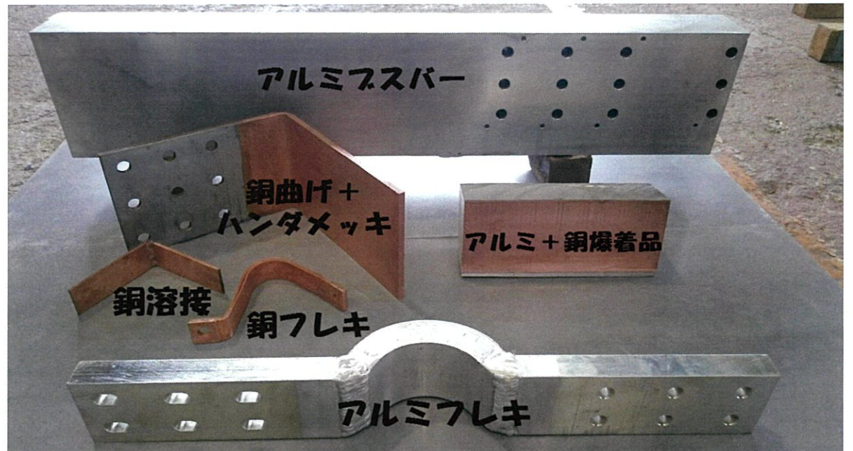
アルミブスバー加工品
